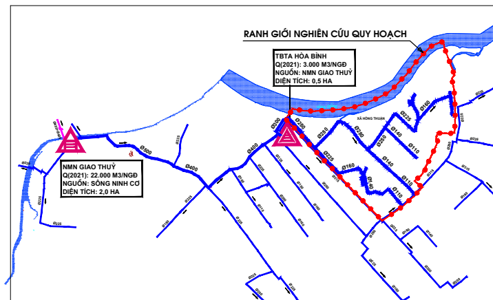
SƠ ĐỒ NGUỒN CẤP NƯỚC ĐÔ THỊ ĐẠI ĐỒNG
